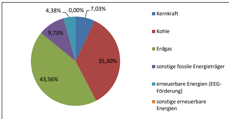
Energieträgermix InfraLeuna GmbH
